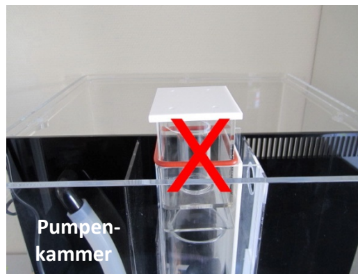
SH1s falsch montiert. Die geschlossene Seite des Eiweißabschäumers zeigt zur Pumpenkammer.
