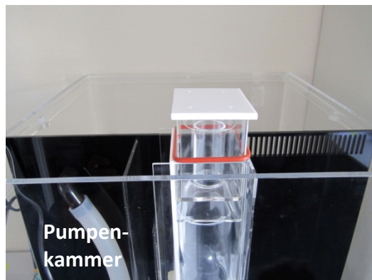
SH1s richtig in der Filterkammer montiert. Die offene Seite des Eiweiß-Abschäumers zeigt zur Pumpenkammer.
